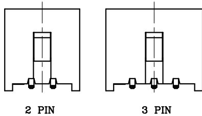
LOCK CONFIGURATION (锁扣位置)
