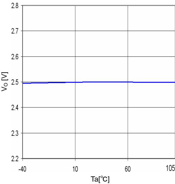
Fig.21 T_a-V_o ( I_o=0mA )
