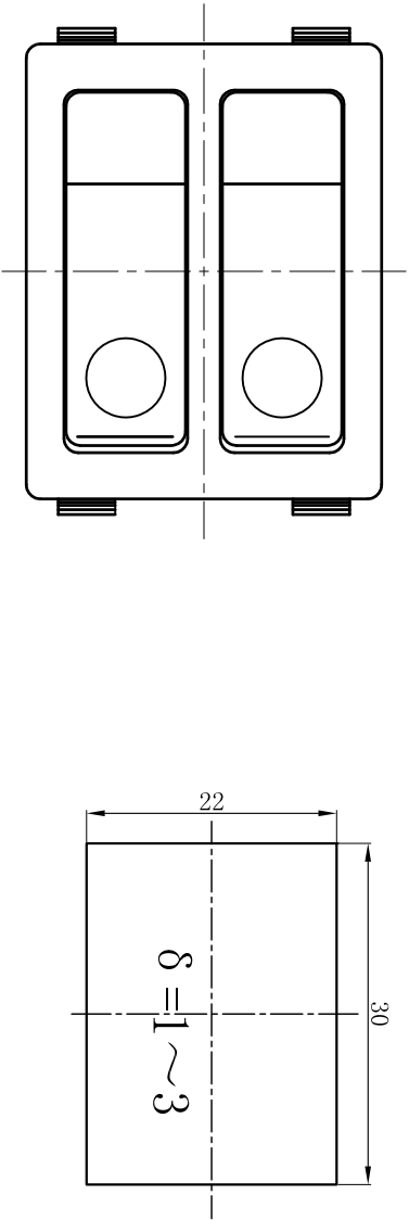
安装面板尺寸 PANEL CUT-OUT
