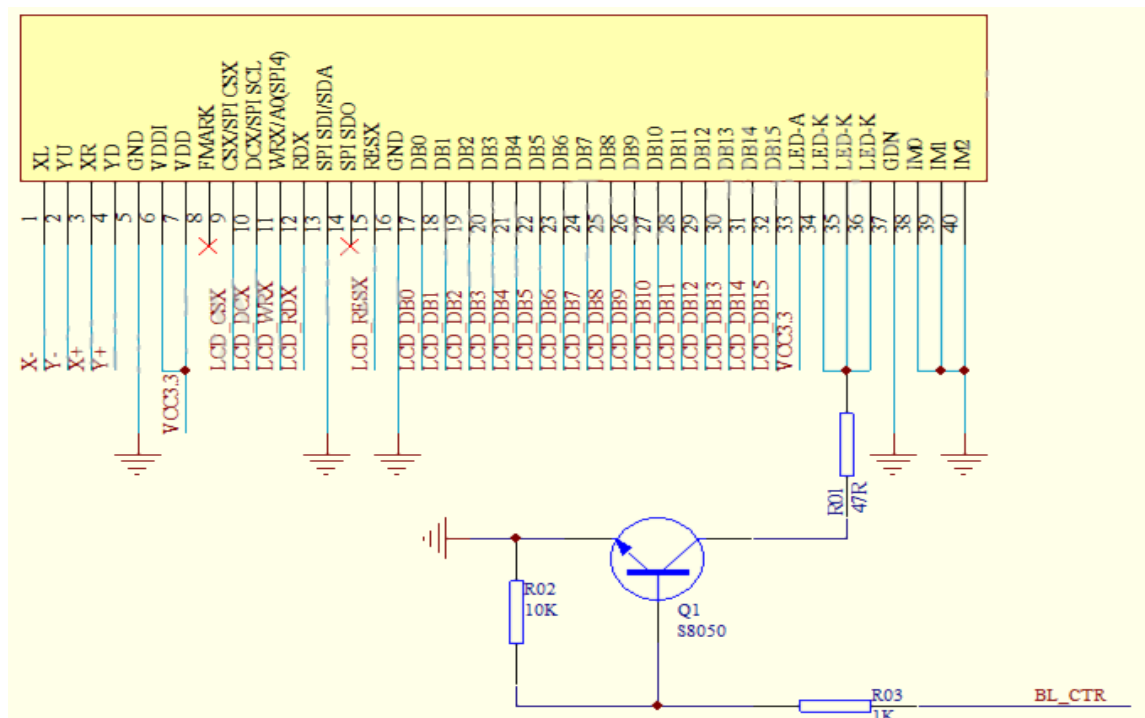
附图 6-1：显示屏 YT240S008_16 位并口参考应用电路
