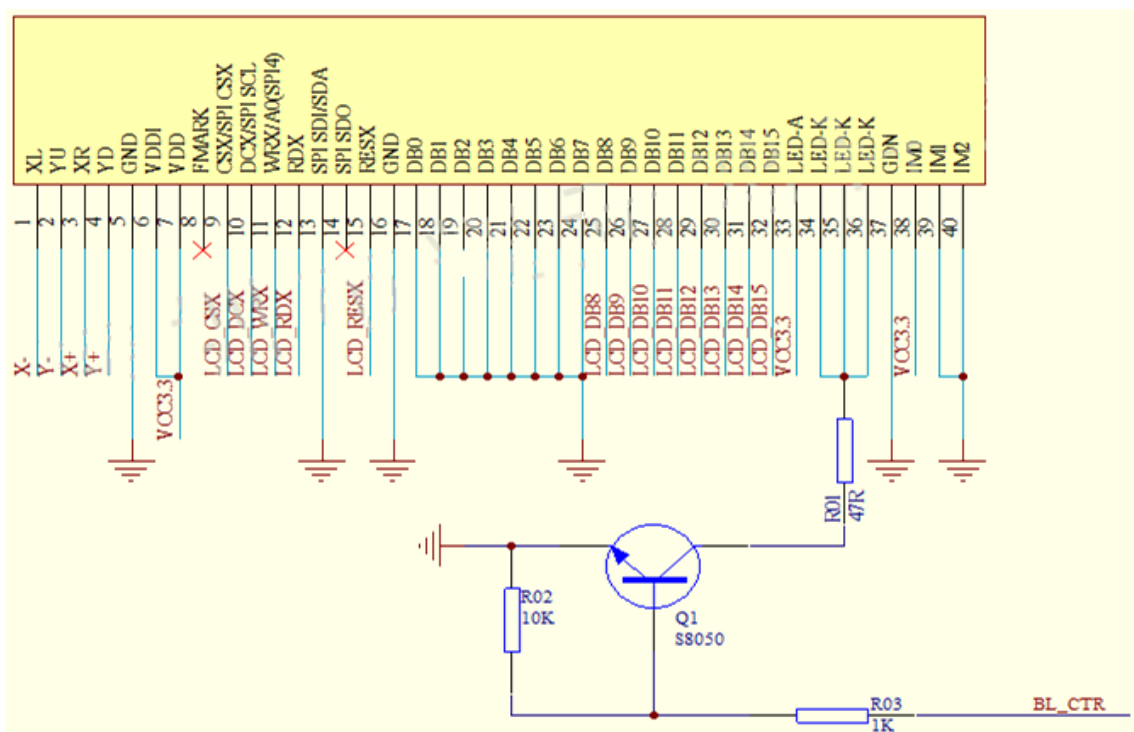
附图 6-2：显示屏 YT240S008_8 位并口参考应用电路
