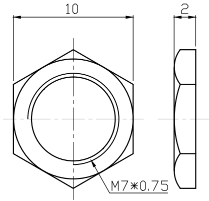
NUT 1pcs
