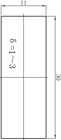
安装面板尺寸 PANEL CUT-OUT
