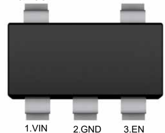
SOT-23-5
