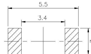
PCB. 焊接图
