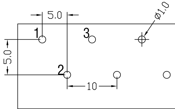
PCB 孔位 1
