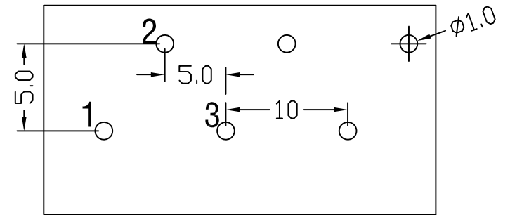
PCB 孔位 2
